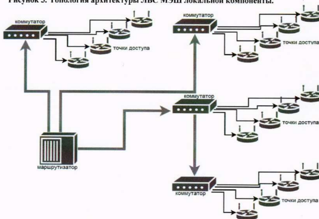
Рисунок 3. Топология архитектуры ЛВС МЭШ локальной компоненты.
